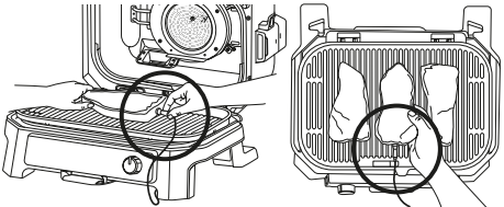
Colocación correcta del sensor. El mango del sensor está totalmente dentro de la unidad.
