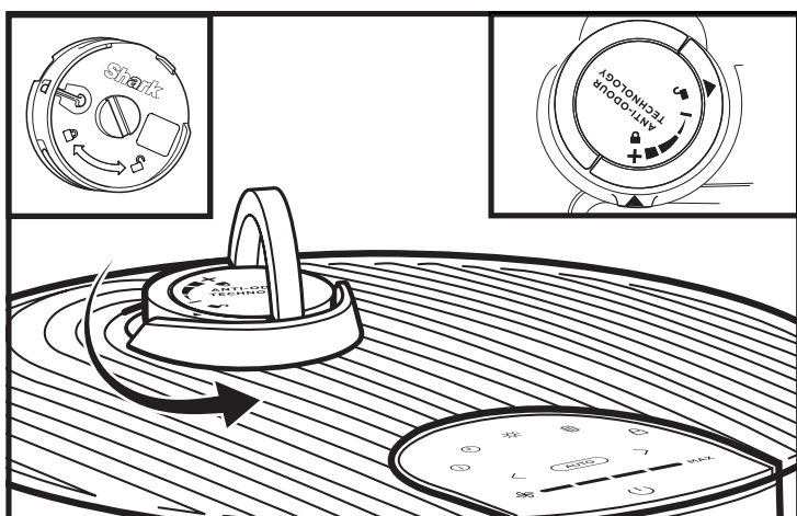
5. INSTALLER LUKTINNSTILLINGSHJULENHETEN
